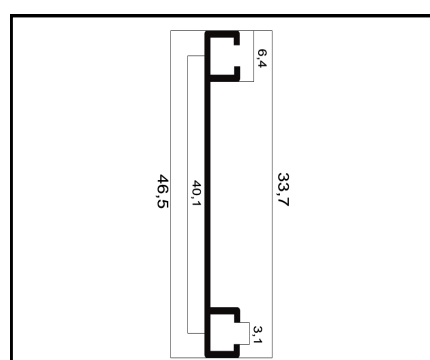
MV-093 TRILHO INFERIOR PESO: 0,150 Kg/m
