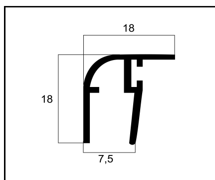
VT-093 CADEIRINHA BOX CANTO PESO: 0,165 Kg/m
