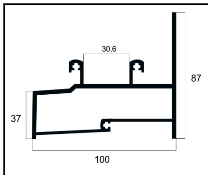
ALG-05 PESO: 1,999 Kg/m
