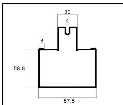
AFE-02 COLUNA PESO: 2,137 Kg/m
