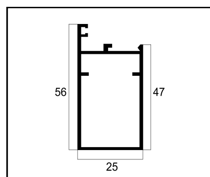
25-504 MONTANTE PESO: 0,634 Kg/m
