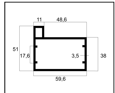
AMT-03 MONTANTE 60 PESO: 0,597 Kg/m
