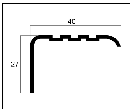
25-116 (ME-13) REMATE DO TRILHO PESO: 0,279 Kg/m
