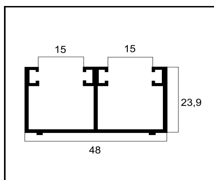
VT10-08 TRILHO INFERIOR DUPLO P/ STANLEY PESO: 0,551 Kg/m
