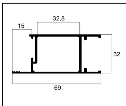
ALG-050 MONTANTE DA FOLHA PESO: 0,880 Kg/m
