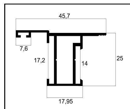
ASU-200 PESO: 0,378 Kg/m
