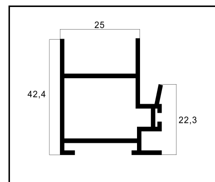
ASU-556 MONTANTE MÃO DE AMIGO PESO: 0,509 Kg/m
