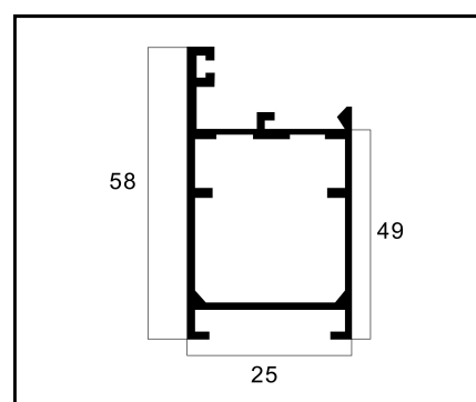
25-023 REQUADRO PESO: 0,638 Kg/m
