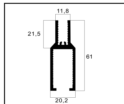
ALH-03 LEITO P/ VIDRO DESLIZANTE (SUPORTE) PESO: 0,759 Kg/m
