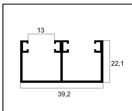
VT10-07 TRILHO INFERIOR DUPLO PESO: 0,437 Kg/m
