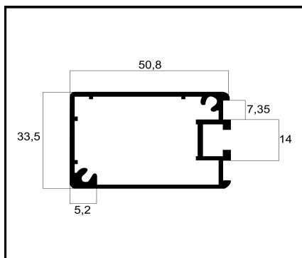
ACG-077 COLUNA PESO: 0,698 Kg/m
