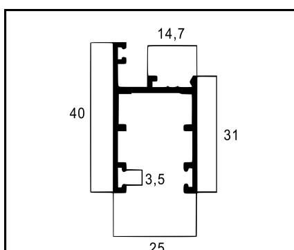
25-014 REQUADRO L-25 PESO: 0,419 Kg/m
