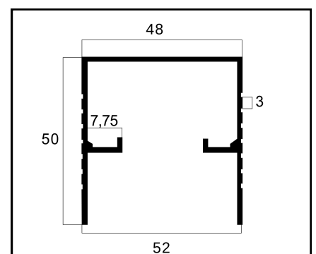
BXS-09 TRILHO SUPERIOR PESO: 0,508 Kg/m
