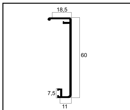
VT10-02 CAPA PESO: 0,297 Kg/m
