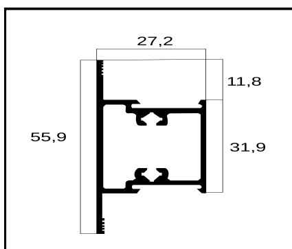
30-017 TRAVESSA PESO: 0,585 Kg/m
