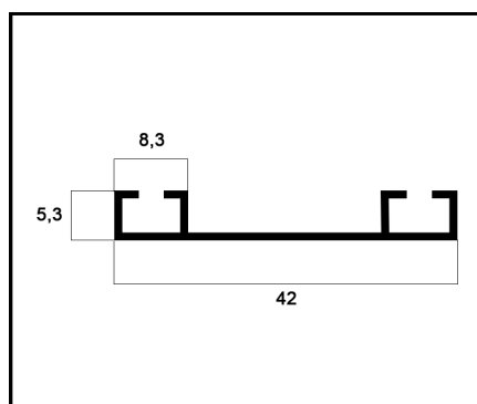
MV-098 PUXADOR PESO: 0,135 Kg/m
