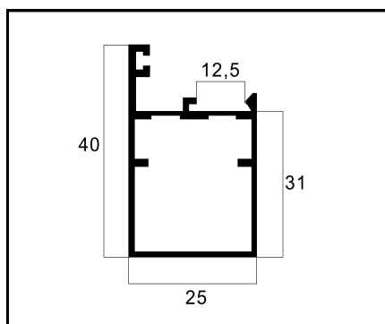
25-011 REQUADRO PESO: 0,469 Kg/m
