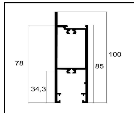
ALG-07 TRAVESSA PESO: 1,311 Kg/m
