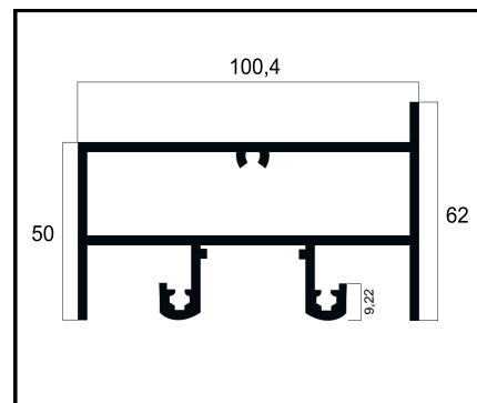
ALG-04 PESO: 1,789 Kg/m
