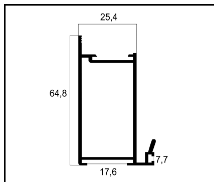
ASU-242 FOLHA MÃO AMIGO EXTERNO PESO: 0,714 Kg/m
