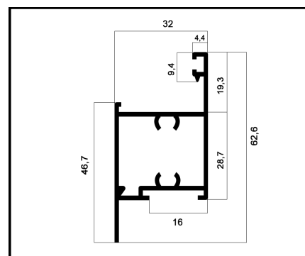
ALG-076 TRAVESSA PESO: 0,597
