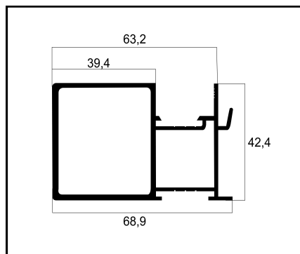
ASU-047 MÃO AMIGO INTERNO C/ REFORÇO PESO: 1,157 Kg/m
