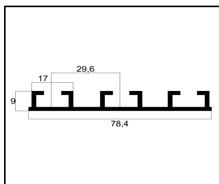
TS-03 TRILHO SUIÇO TRIPLO MAX PESO: 0,340 Kg/m
