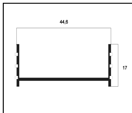
BXS-05 LATERAL PESO: 0,184 Kg/m
