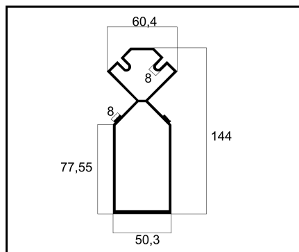
AFE-01 COLUNA CANTO PESO: 2,597 Kg/m
