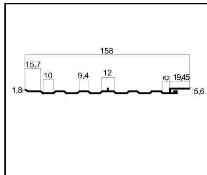
ALB-03 PESO: 0,699 Kg/m
