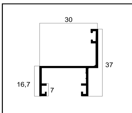
25-02 MARCO P/ MAXIAM AR PESO: 0,339 Kg/m
