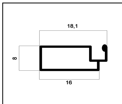
TM-02 PESO: 0,116 Kg/m
