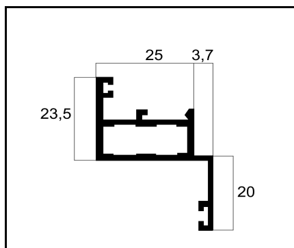
25-05 REQUADRO PESO: 0,469 Kg/m
