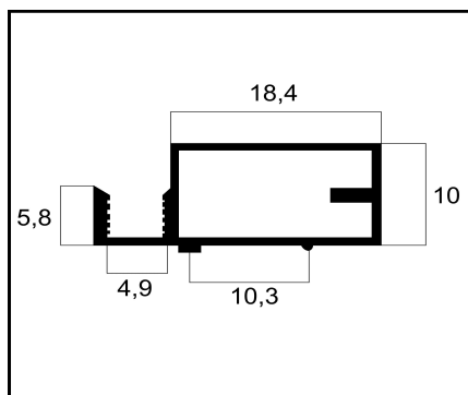
TM-01 TELA MOSQUITEIRO PESO: 0,215 Kg/m
