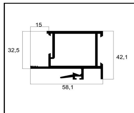
ALG-048 MONTANTE MÃO DE AMIGO LADO DIREITO PESO: 1,021 Kg/m
