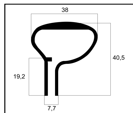
DS-135 PERFIL BORDA PESO: 0,669 Kg/m
