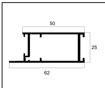
ASU-111 MONTANTE PORTA DE GIRO PESO: 0,687 Kg/m
