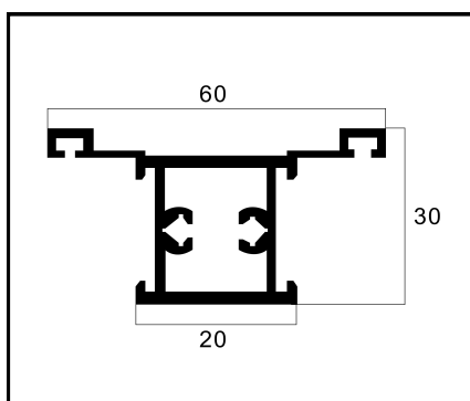
25-07 TRAVESSA PESO: 0,620 Kg/m
