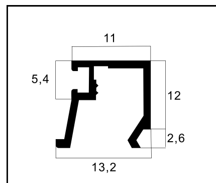
25-201 BAGUETE PESO: 0,110 Kg/m
