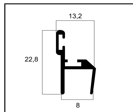
VT-099 CADEIRINHA / BATENTE CENTRAL PESO: 0,166 Kg/m
