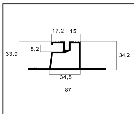
AFE-04 TRAVESSA PESO: 0,976 Kg/m
