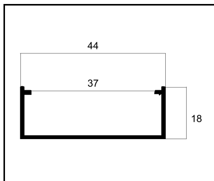
ACG-09 FUNCIONAL/ARREMATE PESO: 0,325 Kg/m
