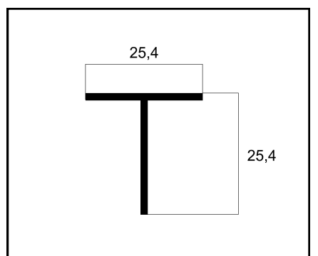
ALB-08 PERFIL "T" 1 X 1,2 MM PESO: 0,186 Kg/m
