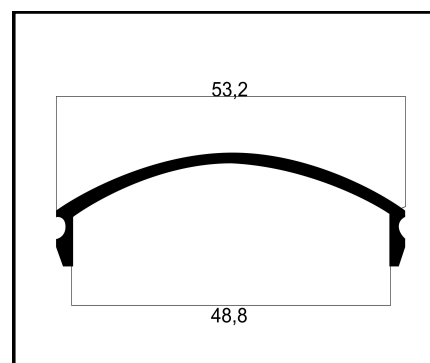
ACG-074 ARREMATE PESO: 0,240 Kg/m
