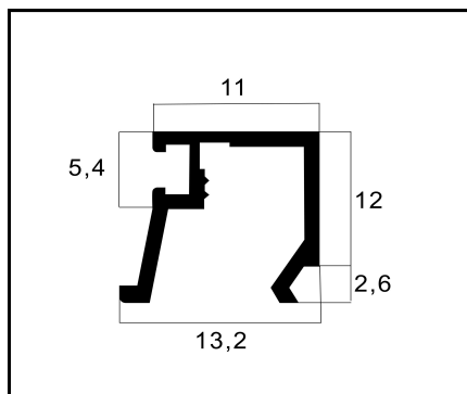
25-01 (BG-01) BAGUETE PESO: 0,101 Kg/m
