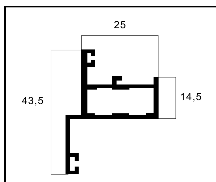
25-205 REQUADRO PESO: 0,437 Kg/m
