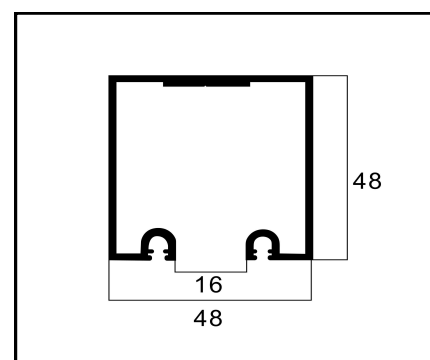
VT10-09 TRILHO SUPERIOR PESO: 0,826 Kg/m
