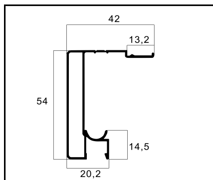
VT-084 TRILHO SUPERIOR PESO: 0,526 Kg/m
