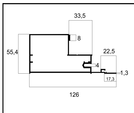
AFE-07 MARCO PARA COLUNA PESO: 1,482 Kg/m
